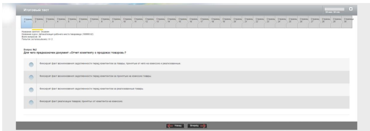
Рис. 4 Пример вопроса
