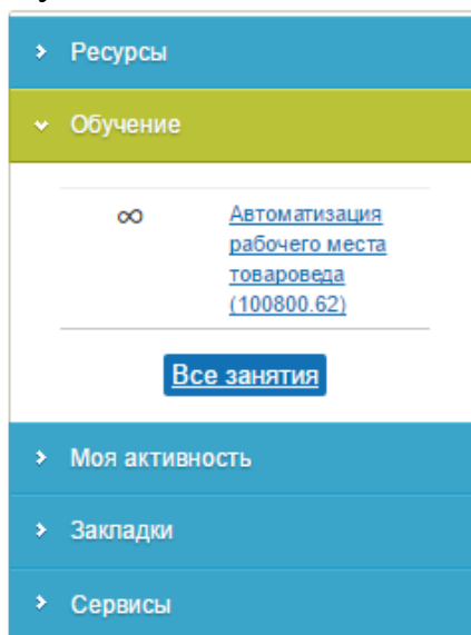
Рис. 3 Все занятия
