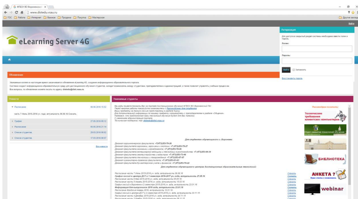
Рис. 1 Начальная страница
