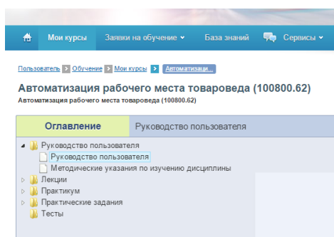
Рис. 4 Оглавление курса
