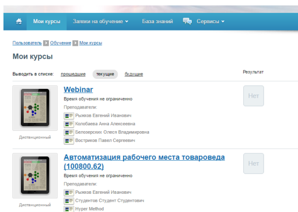
Рис. 2 Мои курсы
