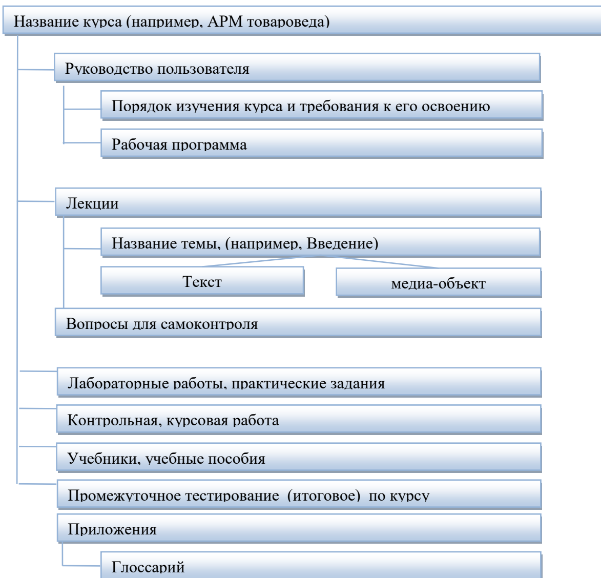
Рис. 5 Структура курса
