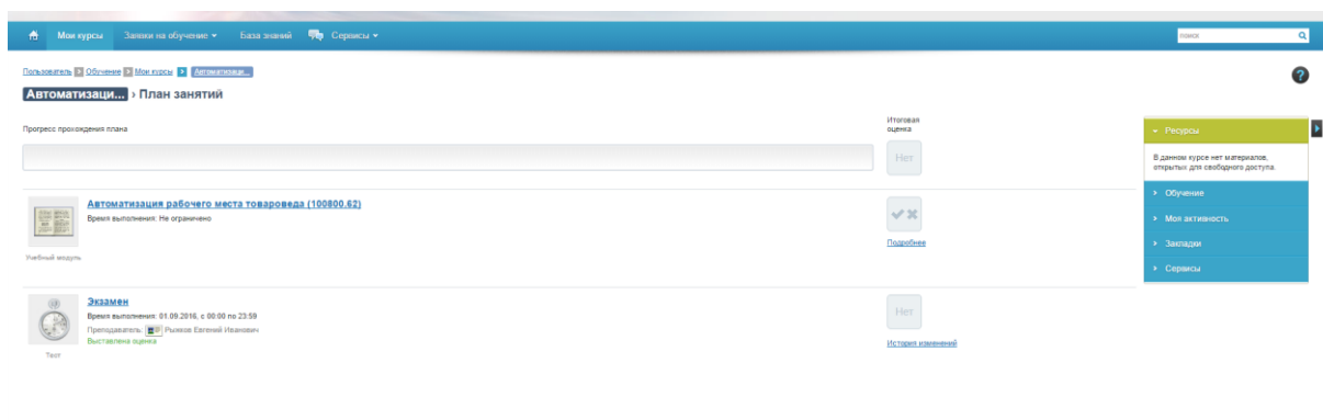
Рис. 6 Назначение занятия
